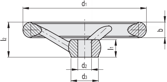
DIN 950-A
